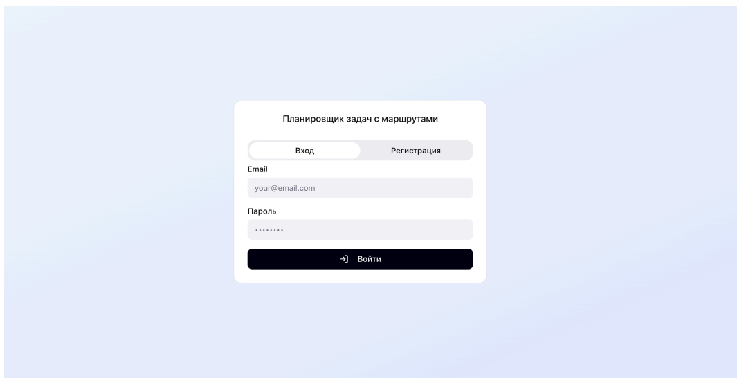
Рисунок 4 – Страница авторизации
