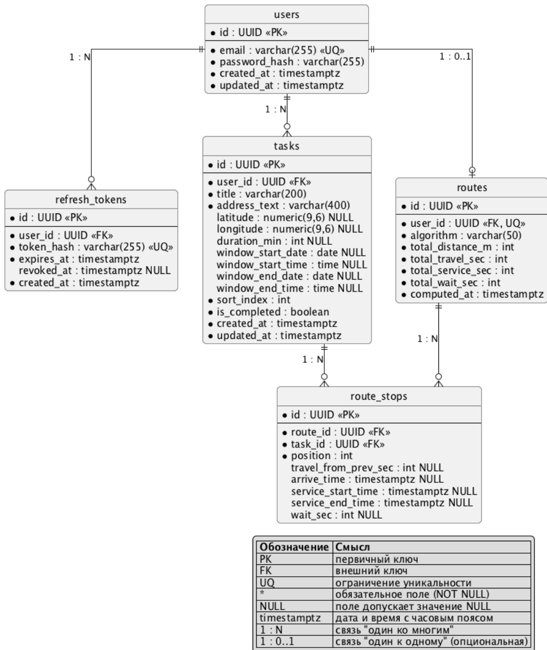
Рисунок 2 – Модель данных
